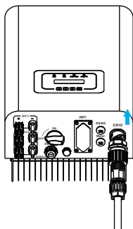
Figura 5.10 Conexão de entrada CA
