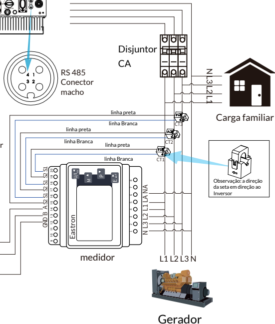
Figura 7.8 Diagrama de conexão do medidor Eastron
