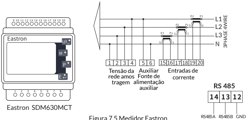
Figura 7.5 Medidor Eastron
